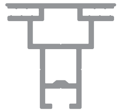
steckkederprofil 50/53 geschlossen
