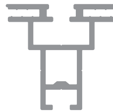
steckkederprofil 50/53
