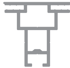
steckkederprofil 50/53 geschlossen
